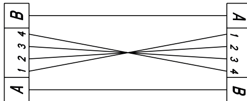
Wiring
